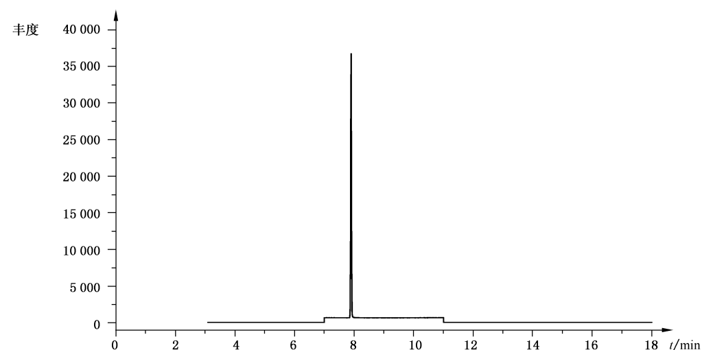
图 A.2 三氯叔丁醇标准品的选择离子色谱图
